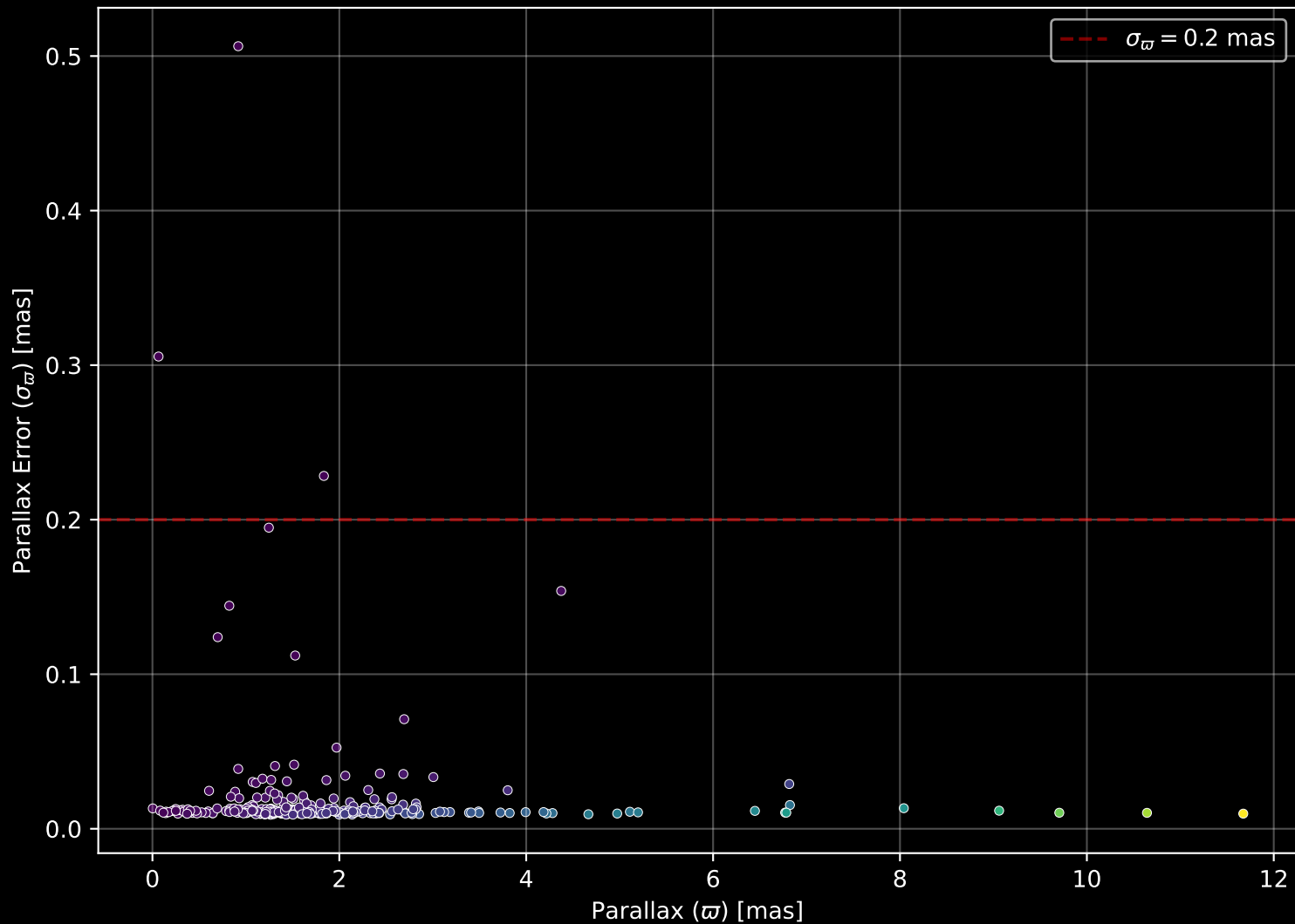
GALAH DR4 Field: [95] Parallax Quality (n= 296)
