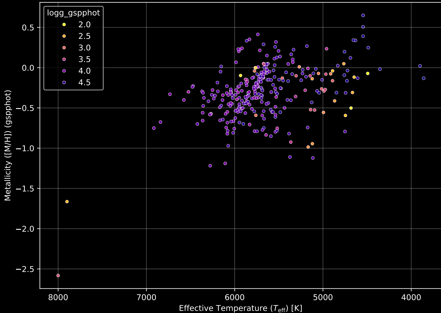
GALAH DR4 Field: [95] Stellar Population Parameters (n= 296)
