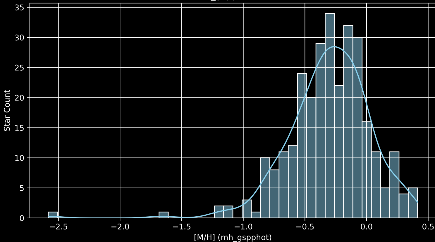
GALAH DR4 Field: [95] [M/H] (mh_gspphot) (n= 294)
